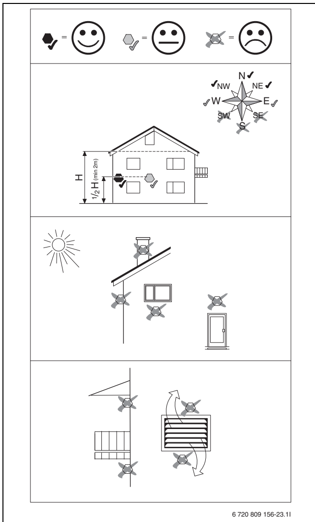
Att. 19 Āra temperatūras sensora izvietošana
