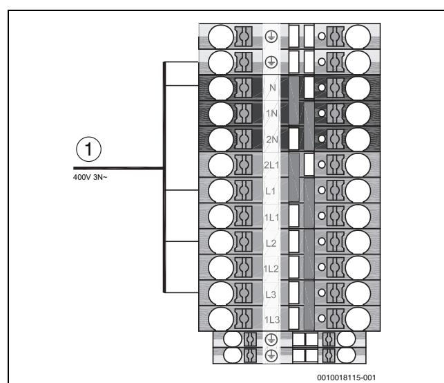
Att. 47 Elektroapgāde piegādes stāvoklī (6 kW, 8 kW, 12 kW, 16 kW)
