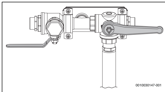
Att. 31 Uzpildes stacija uzpildes pozīcijā
