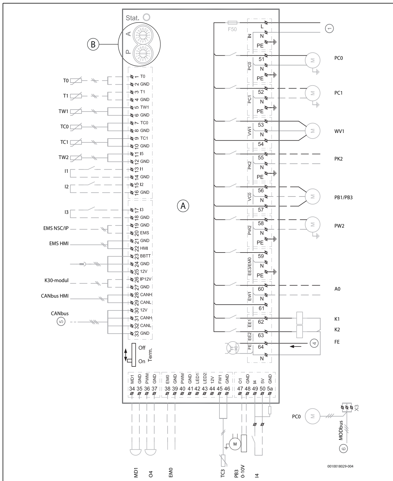
Att. 50 Montāžas vadības plates elektropieslēgumu shēma
