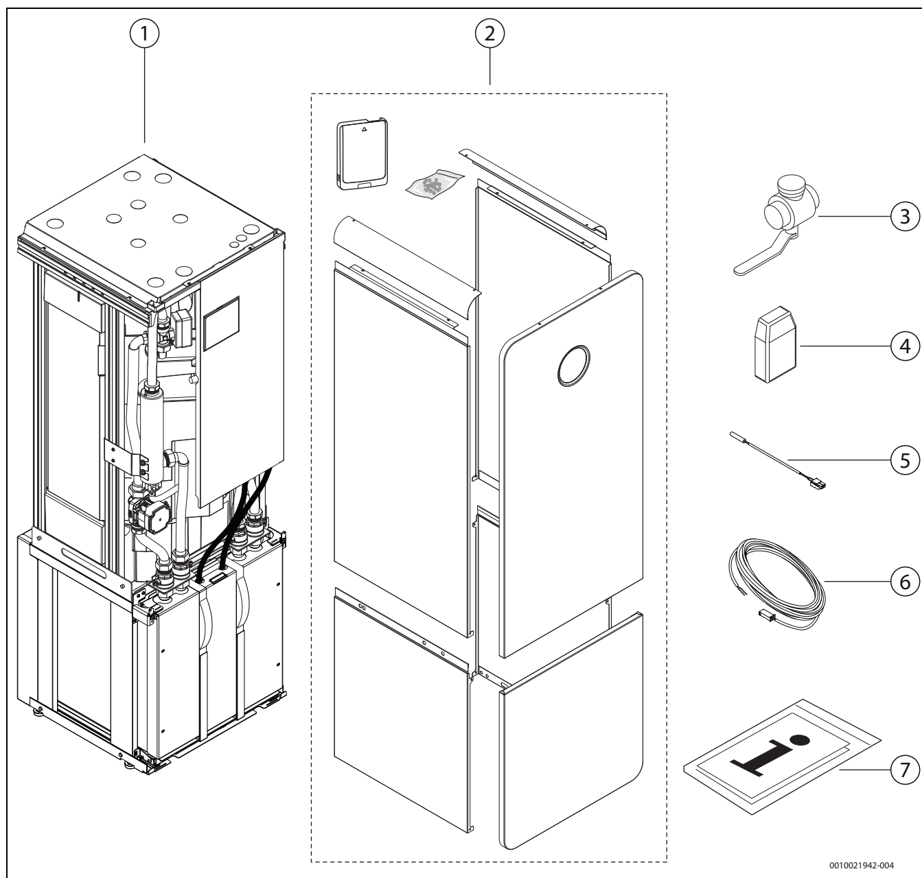
Att. 2 Piegādes komplekts
