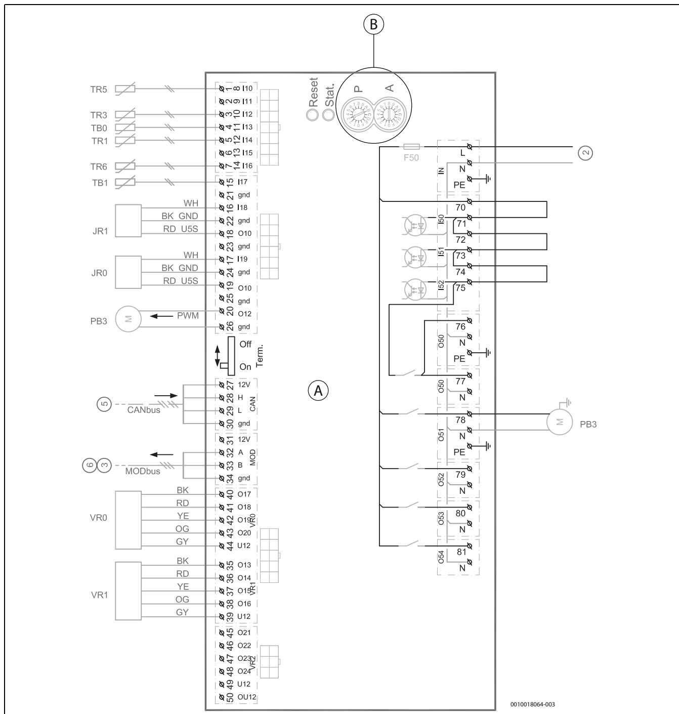
Att. 51 I/O moduļa elektropieslēgumu shēma
