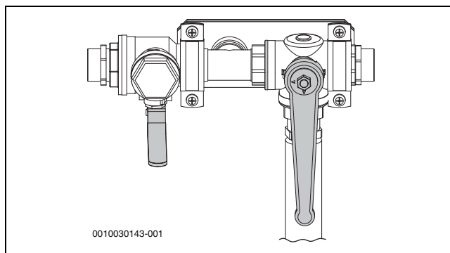
Att. 30 Uzpildes stacija maisīšanas pozīcijā
