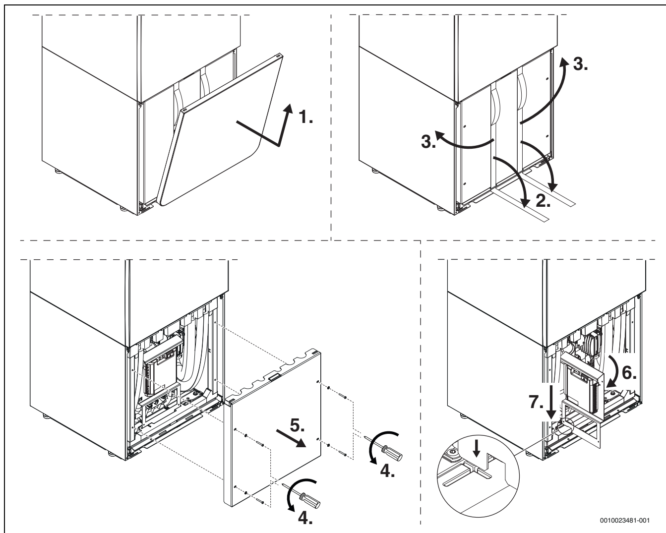
Att. 37 Piekļuve dzesēšanas šķidrums moduļim vienkāršākā apkopē
