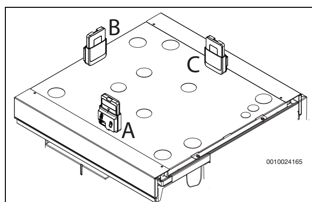
Att. 24 Turētāja piestiprināšana pie augšējā siltumsūkņa pārsega. Bez turētāja attēlā redzams arī turētājā esošais Connect-Key
